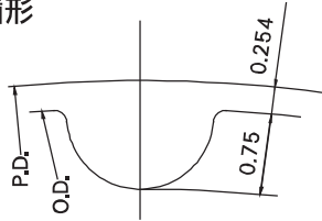
齒形
